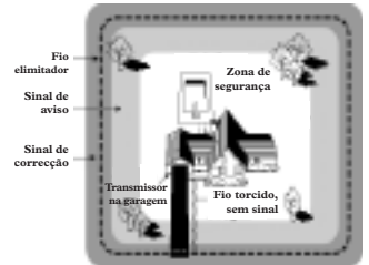
Zona de Segurança Mais Pequena Zona de Aviso Maior
